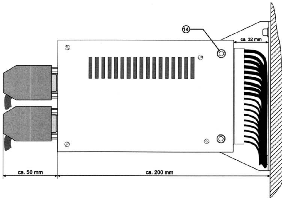
Seitenansicht (bei Wandmontage)
