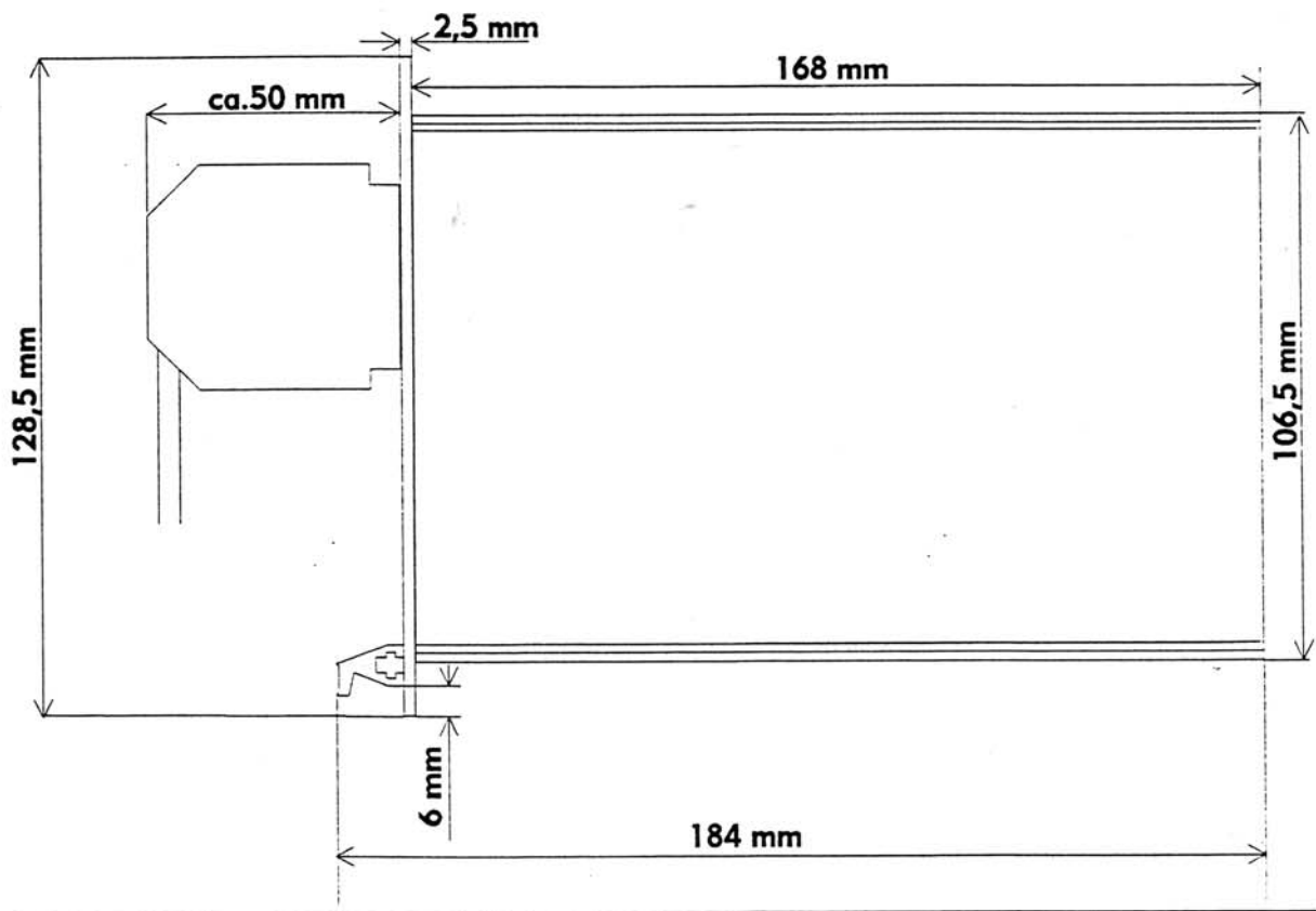
Seitenansicht des 19"-Einschubs mit Gegenstecker vorn Side view 19" Rack with plug-in-type subassembly in front
